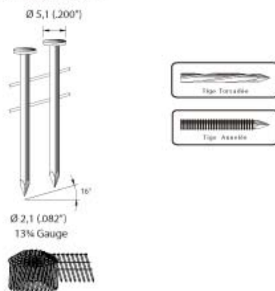
CNW 21 (.082) Bobinage Conique
